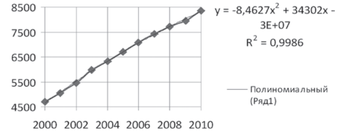
Рис. 4. Полиномиальная зависимость 2-й степени
