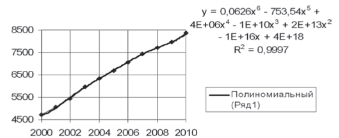
Рис. 6. Полиномиальная зависимость 6-й степени
